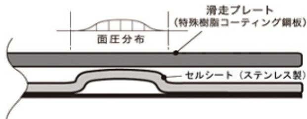
ミューソレーターの構造概念図
