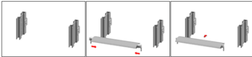
取付手順1
