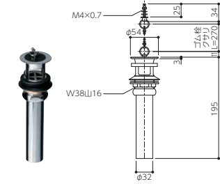
ABH-33T 直管付横穴排水栓 オーバーフロー有りボウル用 (ポップアップ無し)
