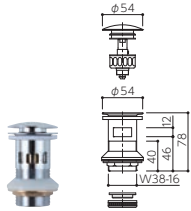
ABH-34M ブラッシュ式ポップアップ横穴排水栓 オーバーフロー付有りボウル用
