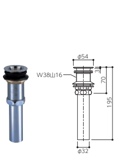
ABH-32 直管付丸鉢排水栓 オーバーフロー無しボウル用
