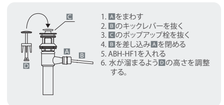
ABH-HF1 ポップアップ用ヘアキャッチャー栓 ●ABH-K280、K250、K210の排水ヘッド部と取り替えてご使用ください。 ●着脱式
