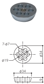
ABH-H39 排水目皿 ●ABH-32、33T対応 ●着脱式
