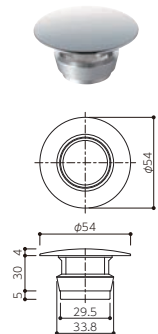
ABH-H341 排水化粧キャップ ●ABH-32対応 ●着脱式
