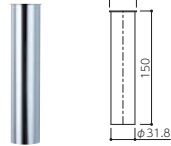
ABH-C 片ツバ直管 ※ABH-34Mとセットでご使用ください。
