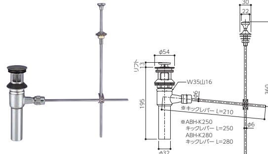
ABH-K210/K250/K280 ポップアップ仕様 オーバーフロー有りボウル用 (ポップアップ有り)
