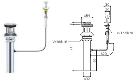
ABH-700W ワイヤー式ポップアップ仕様 オーバーフロー有りボウル用 (ポップアップ有り) ●ポップアップ取付用天板開口：φ15mm ●ヘアキャッチャー付き
