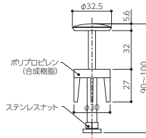
ABH-HF1 ポップアップ用ヘアキャッチャー栓 ●ABH-K280、K250、K210の排水ヘッド部と取り替えてご使用ください。 ●着脱式
